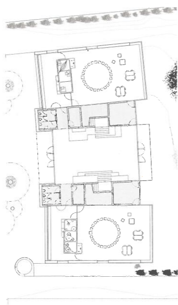
Erdgeschoss Kindergarten
