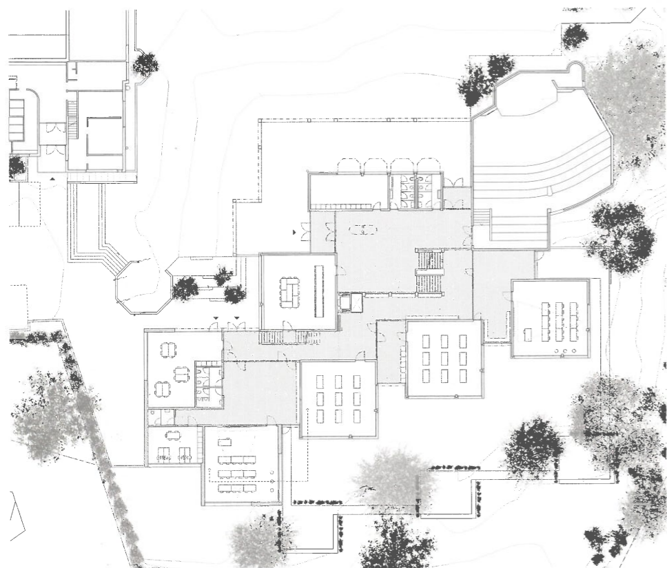
Erdgeschoss Schulhaus
